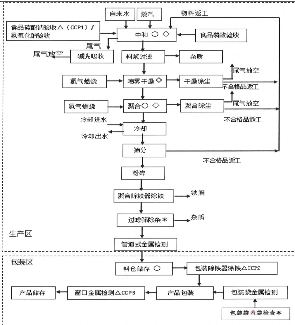
图 3-1 生产工艺流程图
